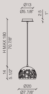
HOLE Ø20
