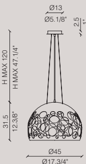
HOLE Ø45
