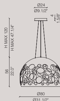
HOLE Ø80
